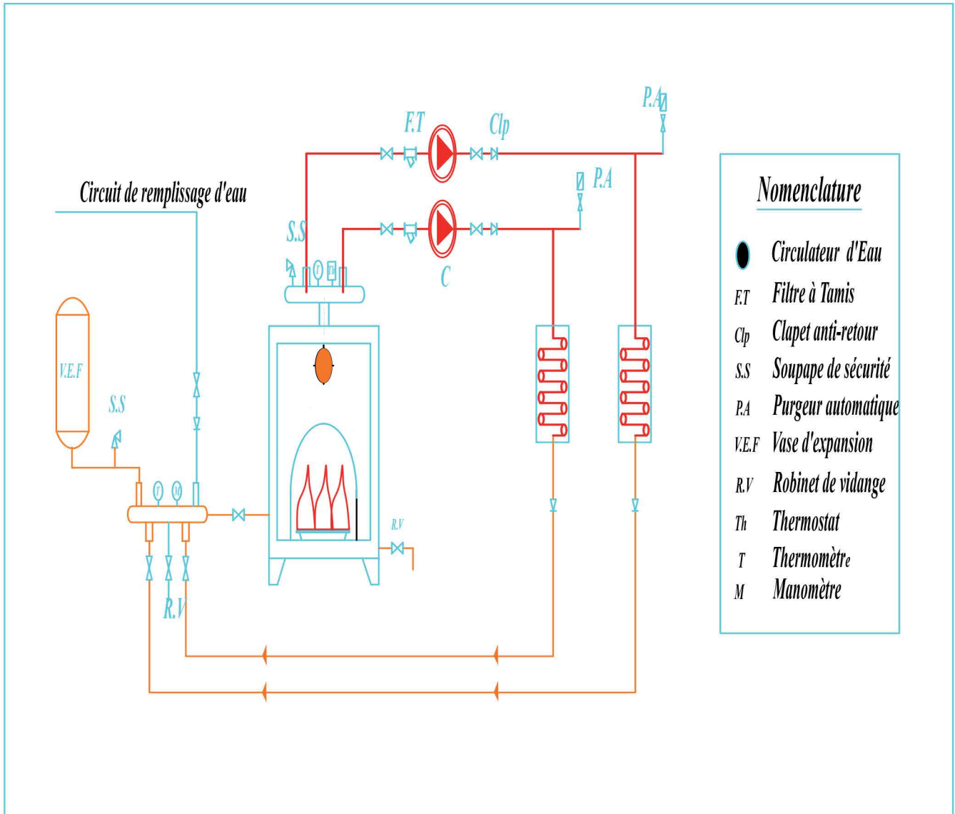
Schéma de principe hydraulique Installation type / avec vase d'expansion fermé
