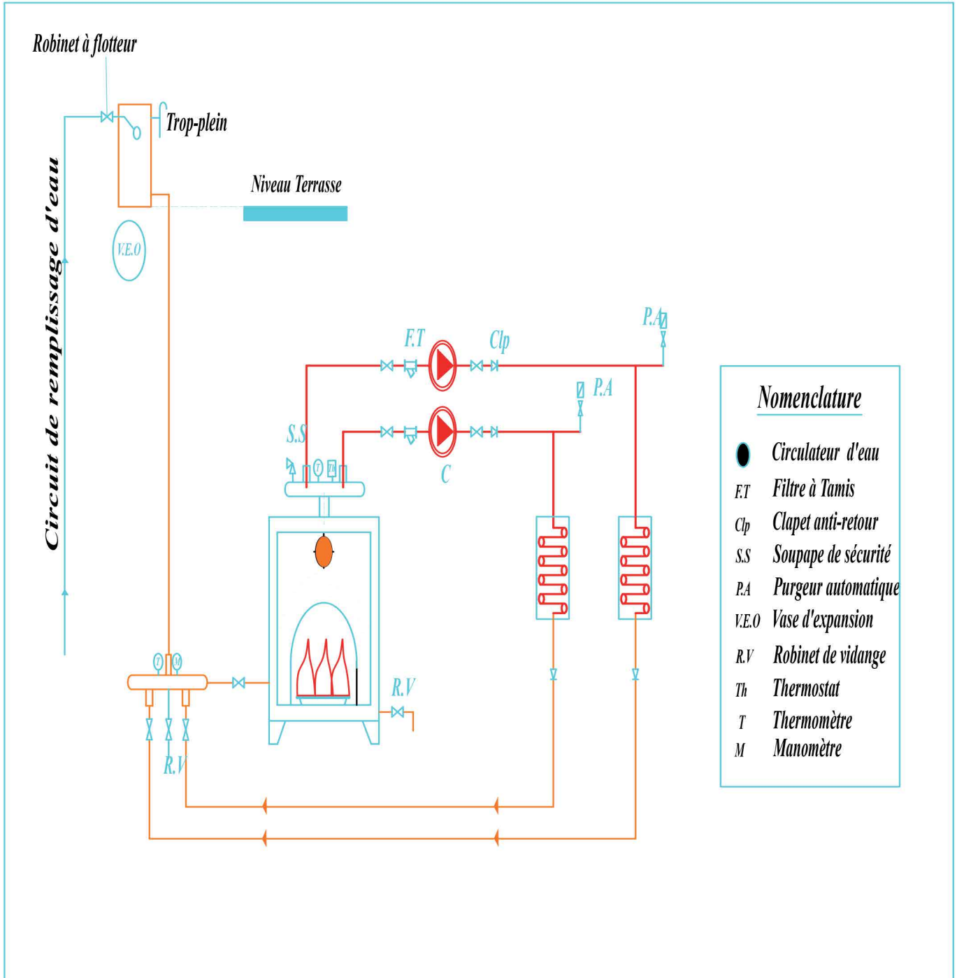
Schéma de principe hydraulique Installation type / avec vase d'expansion ouvert
